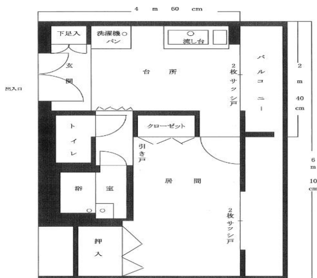
A B棟間取り
